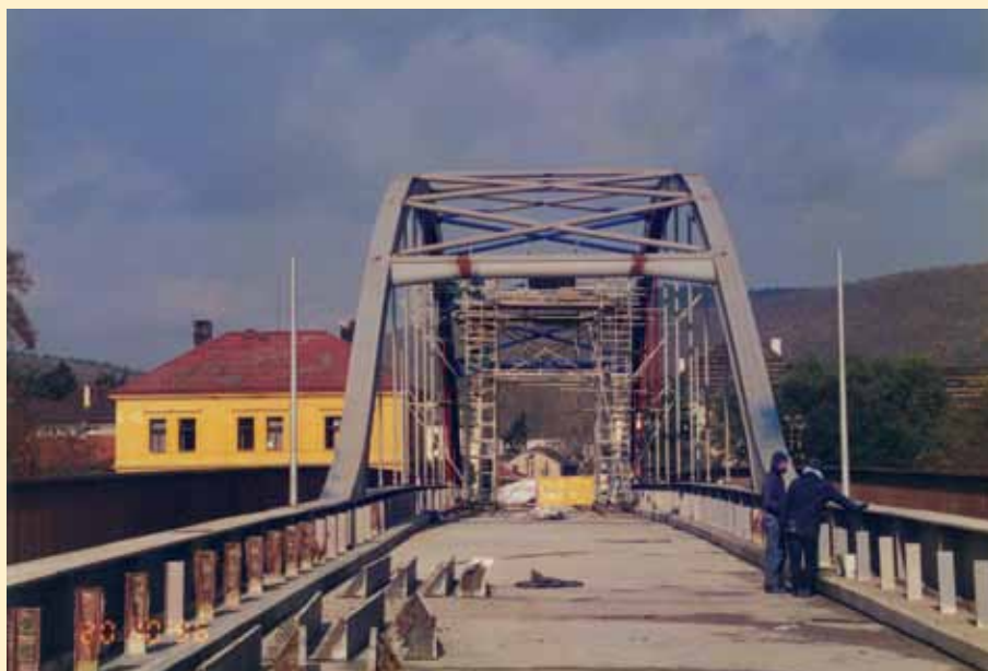
Říjen 1996 – dokončovací práce na mostě (nátěry, izolace, vozovky, chodníky)
