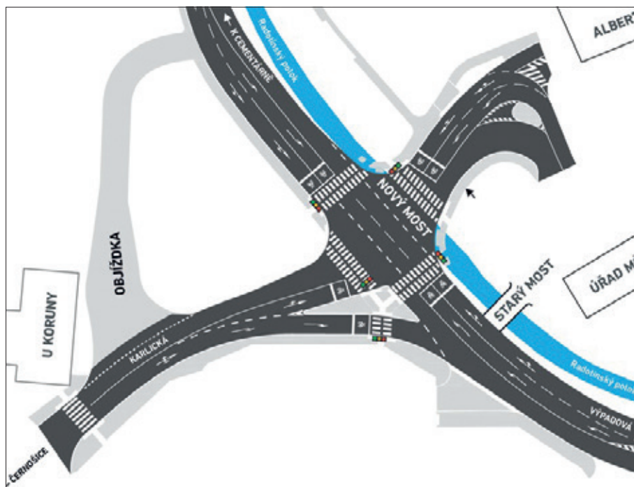
Půdorys vznikající nové křižovatky v Radotíně
